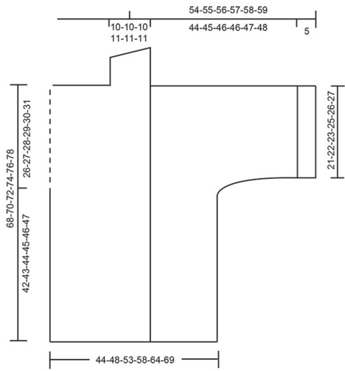
Diagram til DROPS 222-36
